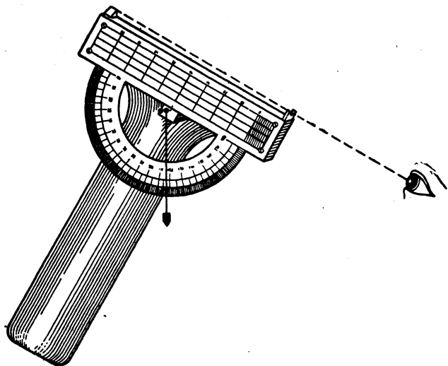
Рис. 34. Ручной высотомер.
