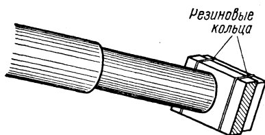
Рис. 22. Коробка на окулярном конце телескопа для фотопластинки.
