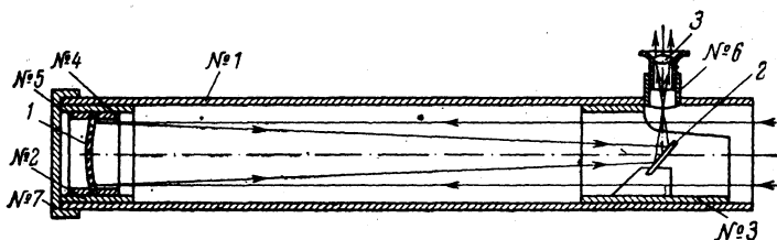
Рис. 6. Схема гелиоскопа.
