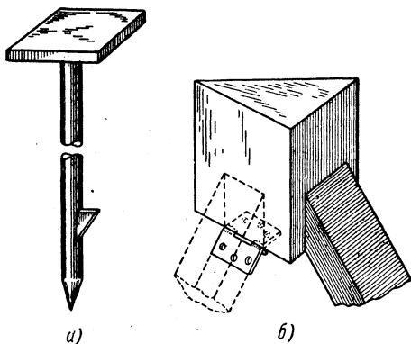
Рис. 11. Штатив в виде переносного столба и призма переносной треноги.
